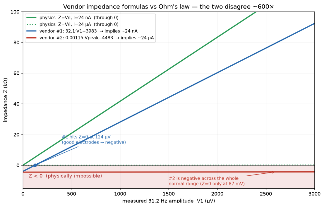
图 2: 厂商两个阻抗公式与欧姆定律 Z = V/I (过原点) 的对比。两个公式都带 负载距 (好电极会算出负阻抗, 粉色不可能区), 且其斜率反推出的注入电流相差约 600\times (公式 #1 \Rightarrow \sim 24 \text{ nA} , 公式 #2 \Rightarrow \sim 24 \mu\text{A} ), 二者不可能同时成立。
