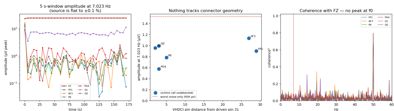
图 4: 左: f_0 处的 5s 分窗幅度。信号源是平的, 悬空通道在 1\mu\text{V} 附近游走, 与之无关。中: 幅度对 VHDCI 引脚距离。右: 与被驱动通道的幅度平方相干, f_0 处没有峰。
