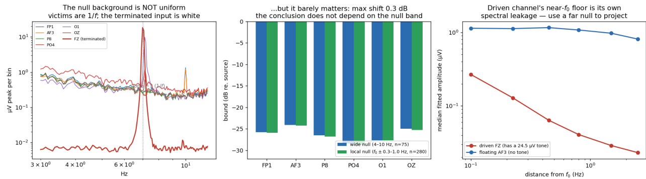
图 5: 左: 零分布带内的背景。每个悬空通道都服从 1/f ; 唯一那个终接通道在同一段里是白的 (斜率 +0.21 )——一个正常偏置的输入本该就是这样。中: 用宽零分布算的上界, 与紧贴 f_0 的局部零分布对比。右: 被驱动通道的拟合幅度对「距 f_0 的距离」——单调衰减, 那是它自身音调的谱泄漏, 在不携带音调的通道上不存在。
