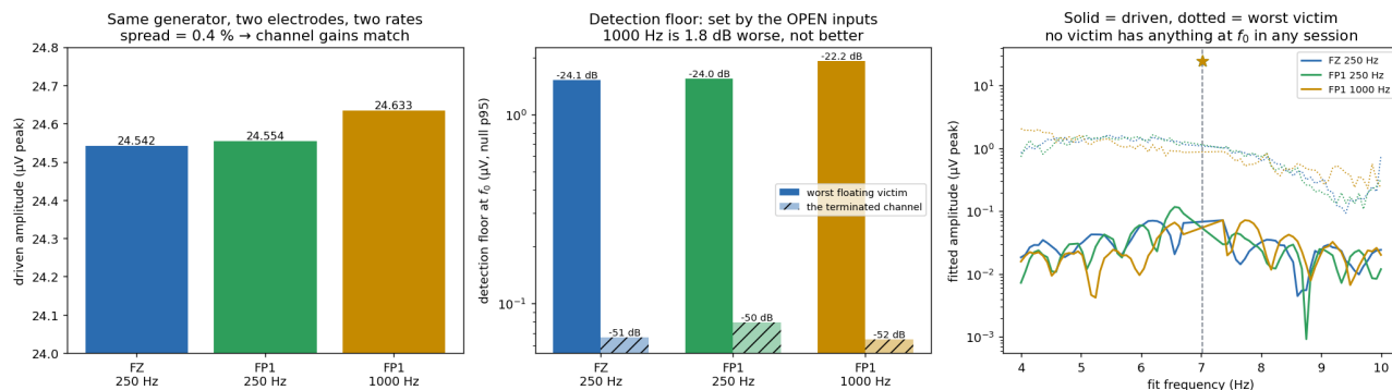
图 6: 左: 三次测量的被驱动通道幅度, 总离散 0.37%。中: 检出下限, 分成终接通道 (斜纹) 和最差悬空通道两部分——两者之间约 27 dB 的差距, 就是「输入不接」这件事的全部代价。右: 三次测量的扫频曲线叠在一起, 实线是被驱动通道, 虚线是该次最差的被测通道。每一条虚线都平滑地穿过 f_0 。
