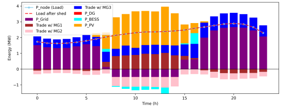
(d) Active Power MG4
