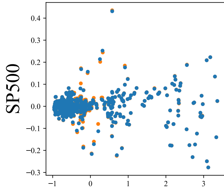
PCA
