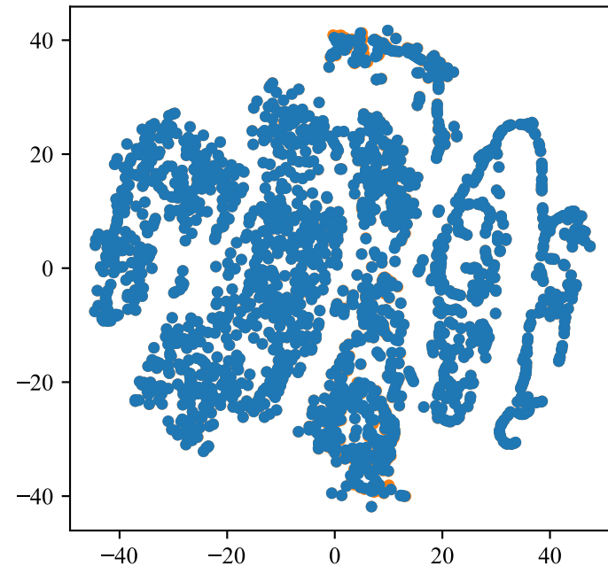
t-SNE
