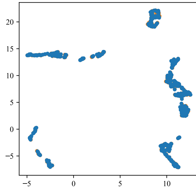
UMAP
