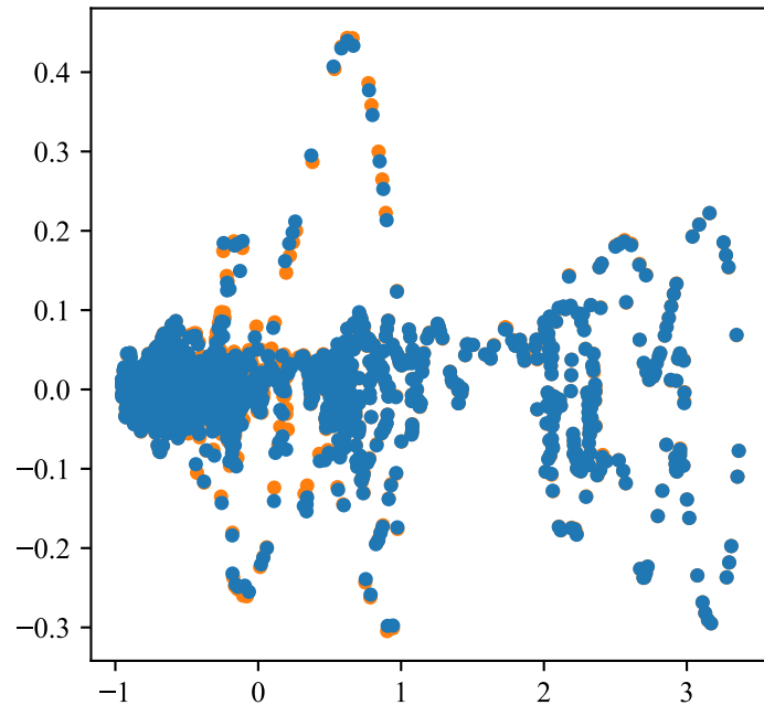
PCA
