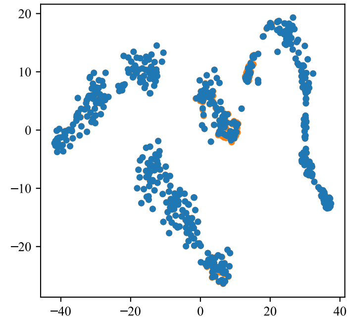
t-SNE
