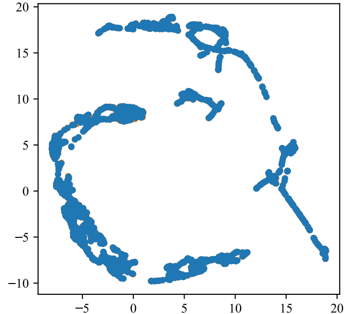
UMAP
