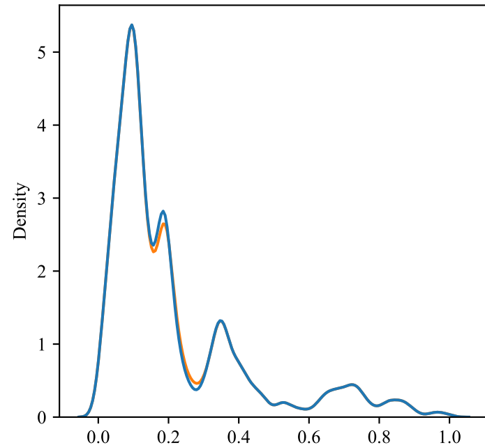
KDE
