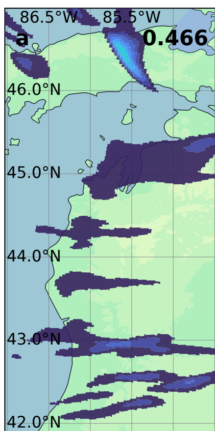
HRRR
