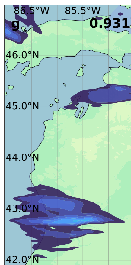
LESNet-B
