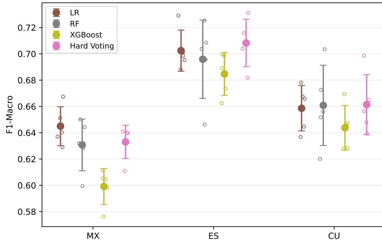
F1-Macro
