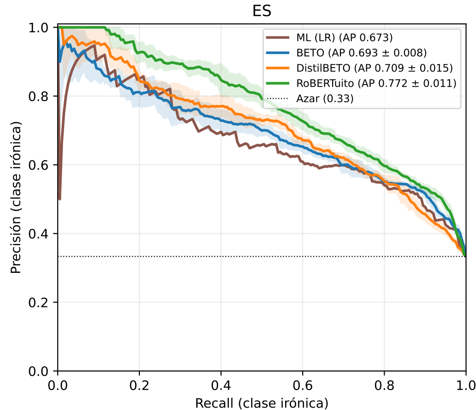
Curva Precision-Recall en el test oficial (Transformers: media \pm d.e. de 5 semillas)
