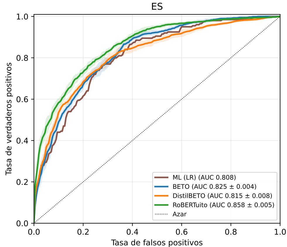
Curva ROC en el test oficial (Transformers: media \pm d.e. de 5 semillas)
