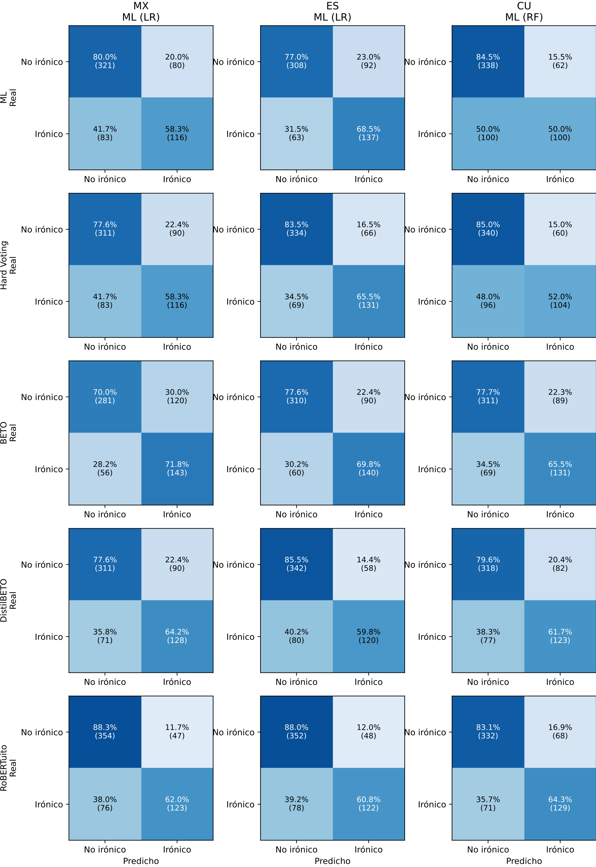
Matrices de confusión en el test oficial (% por clase real)
