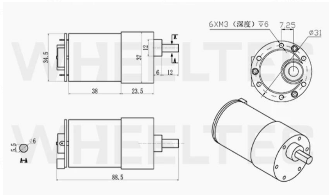
图 3-2 MG540 电机机械参数
