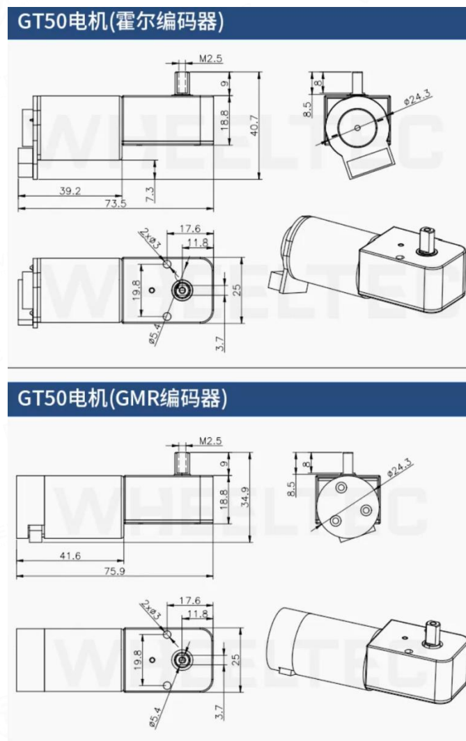
图 7-2 电机机械参数图示
