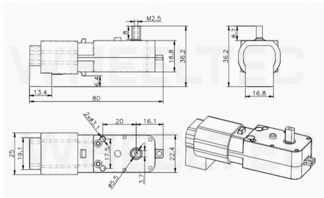
图 8-2 电机机械参数图示
