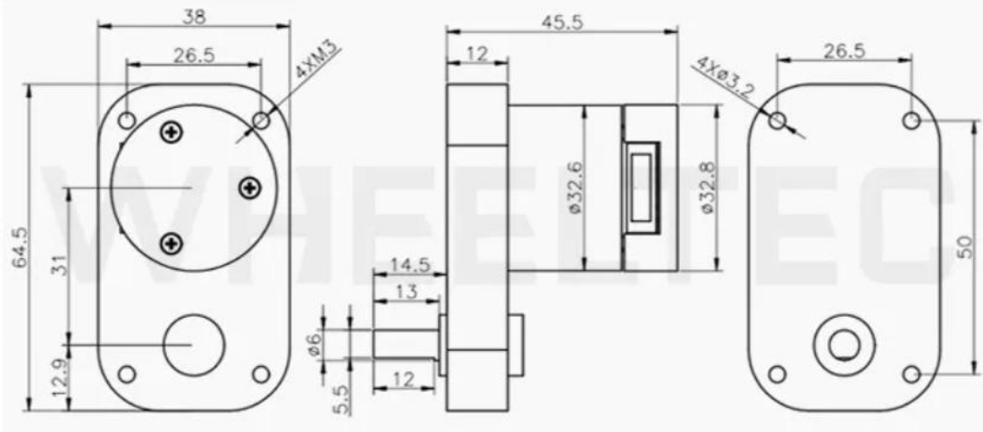
图 2-2 电机机械参数图示
