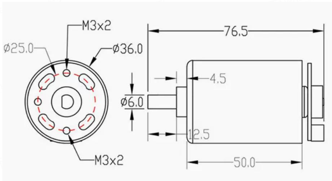
图 6-2 电机机械参数图示
