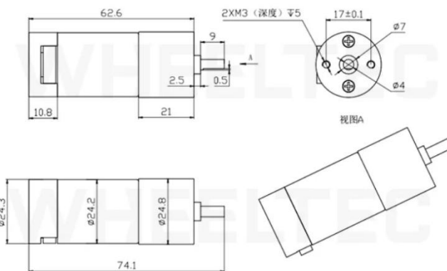
图 5-2 电机机械参数图示
