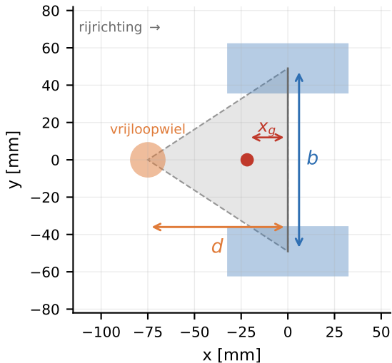
bovenaanzicht: steundriehoek
