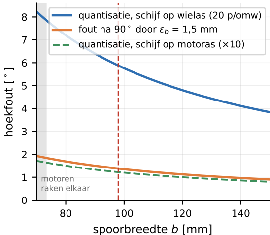
hoekfout van de odometrie
