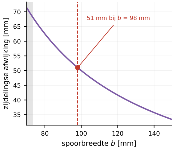
koersdrift over 1 m bij 1 % wielverschil
