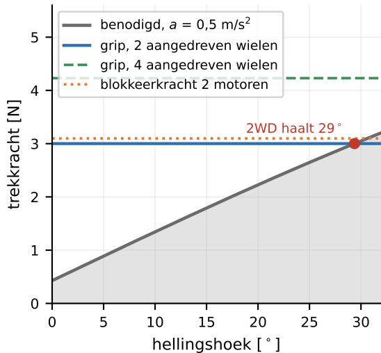
trekkrachtbudget
