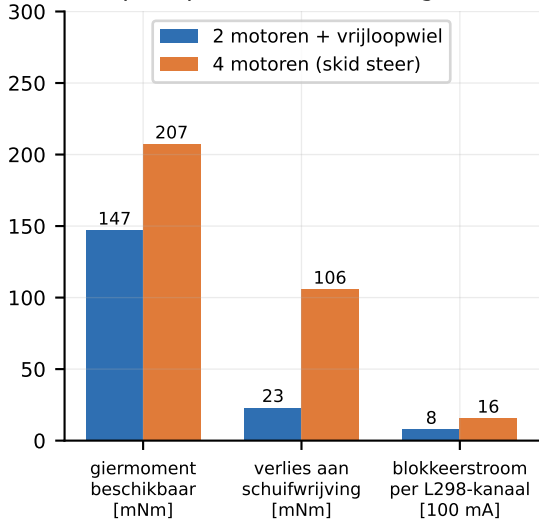
draaien op de plaats, en belasting van de L298
