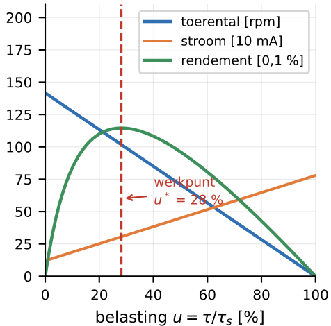
motorkarakteristiek bij U_m
