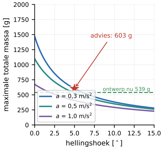
wat twee motoren duurzaam trekken
