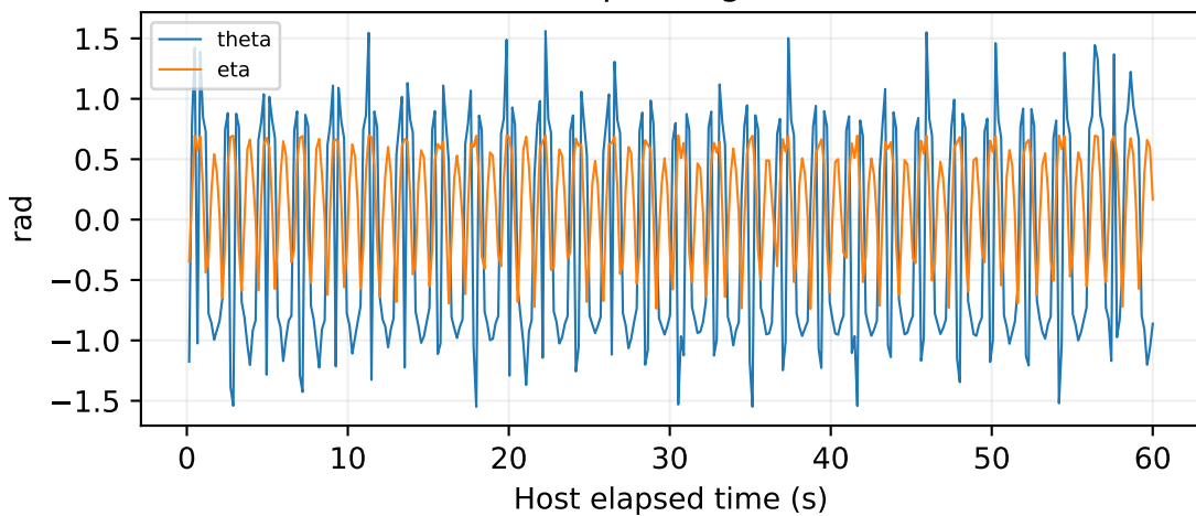
Ellipse angles
