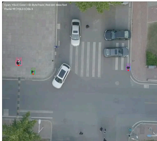
色付きの枠と ID: ByteTrack / 赤点: 足元の座標
