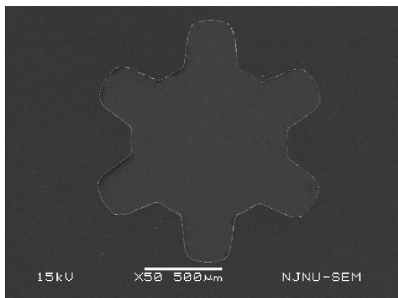
(a) 单联硅齿轮
