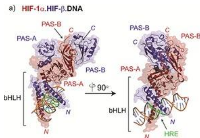
Рисунок 1 – Изображения рентгеновской кристаллической структуры гетеродимера HIF-1α/β bHLH-PAS в комплексе с ДНК
