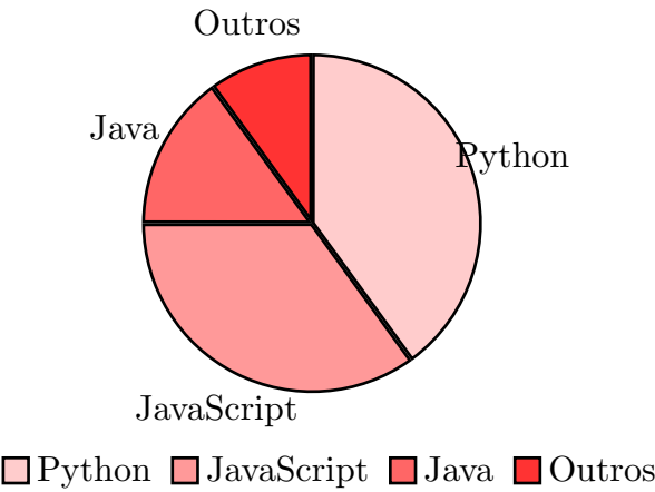
Figura 3 – Distribuição linguagens
