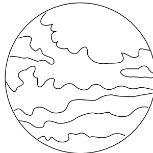
fcPlanetC
