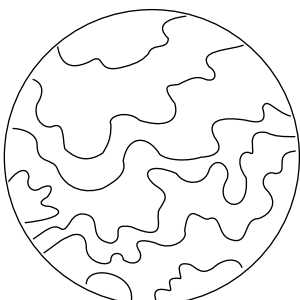
fcPlanetG
