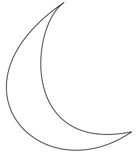
fcMoon
