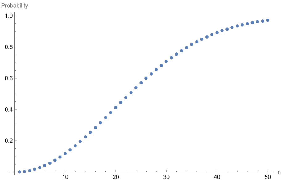
图 1 概率随 n 的变化 / Probability versus n
