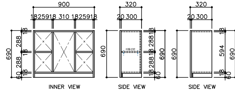
후드장/제작도면
