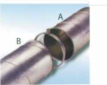
束带连接 Loincloth connect
