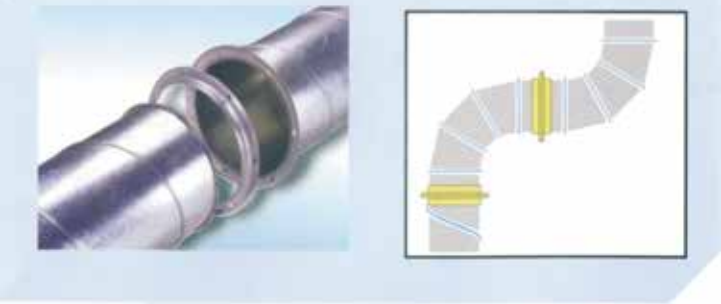
角钢法兰连接 Angle iron flange connect
