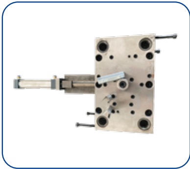
共板卡条连续模具 TDF Cleat
