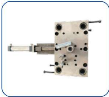
共板卡条连续模具 TDF Cleat
