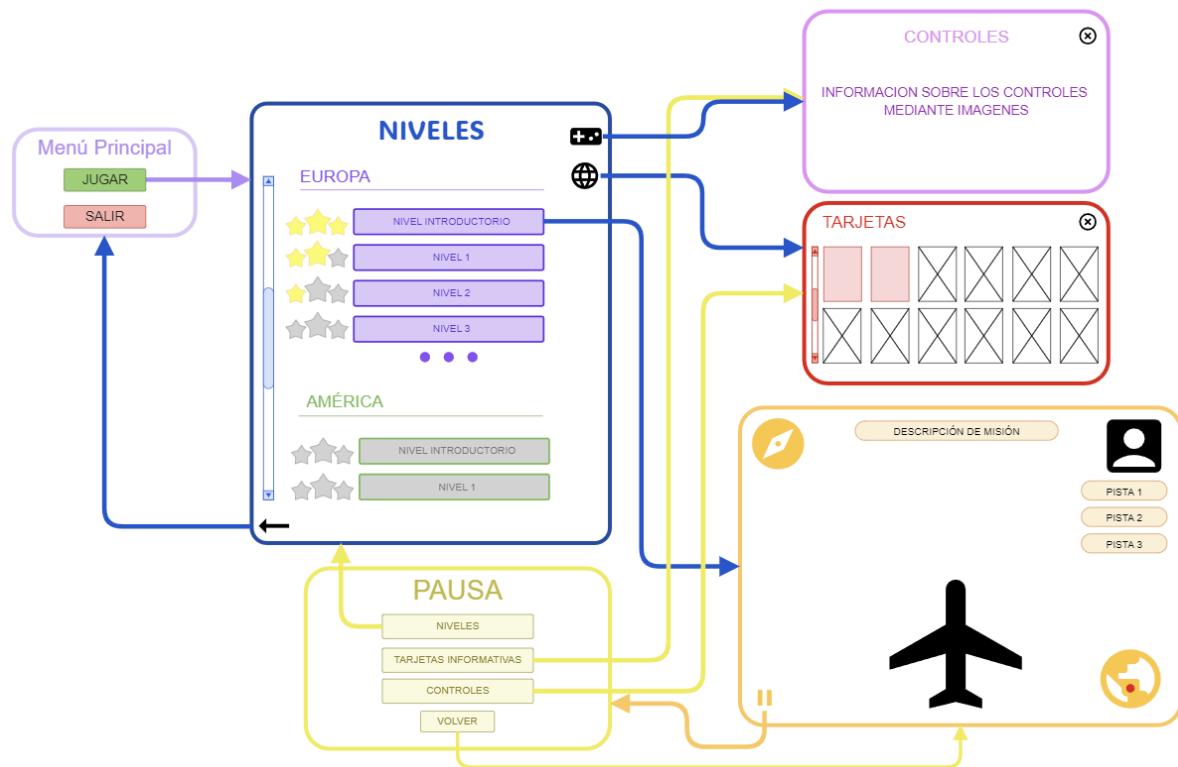
Imagen 10. Diagrama de flujo de juego de todos los menús e interfaces.
