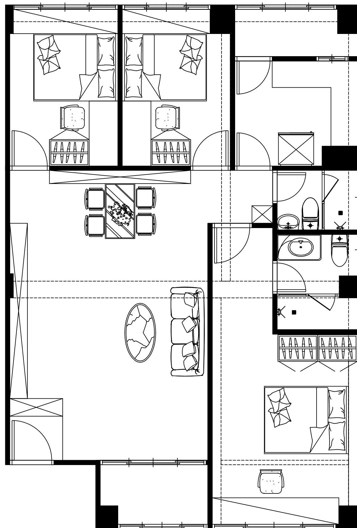
設計平面圖B
