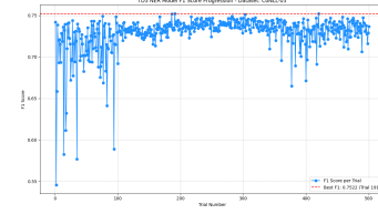
Fig. 9. CONLL TD3
