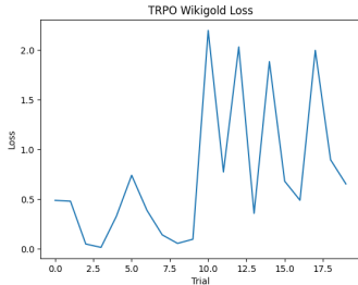
Fig. 8. TRPO WG
