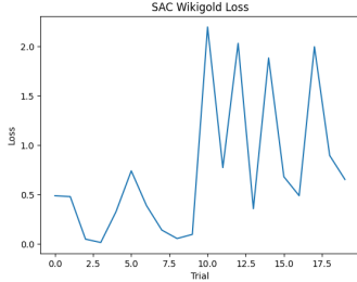
Fig. 7. SAC WG
