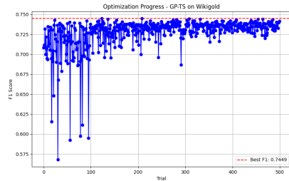
Fig. 3. Wikigold F1 Score Evolution via GP-TS
