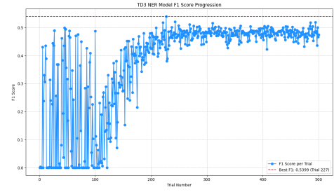
Fig. 4. Wikigold F1 Score Evolution via TD3
