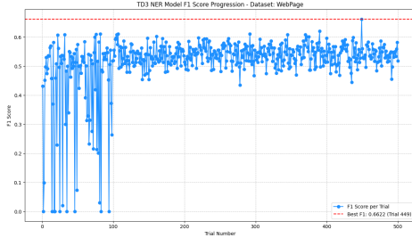
Fig. 2. Webpage F1 Score Evolution via TD3
