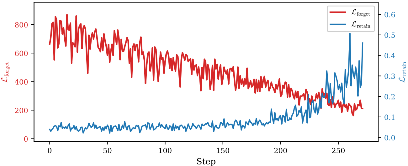
MUSE Books — Llama-2-7B: PDU (HM = 0.602)
