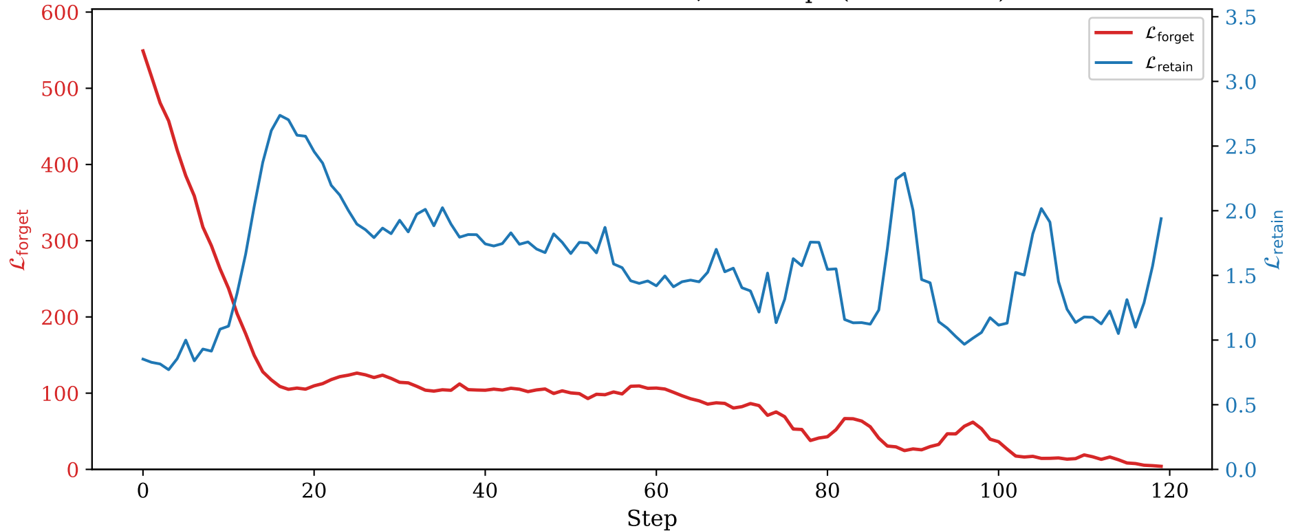
MUSE News — Llama-2-7B: PDU, 120 Steps (HM = 0.581)
