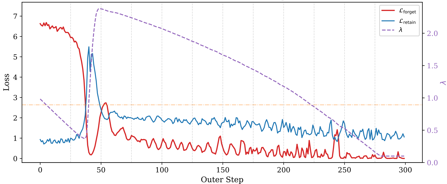
MUSE News — Llama-2-7B: BLADE, 300 Steps (HM = 0.542)
