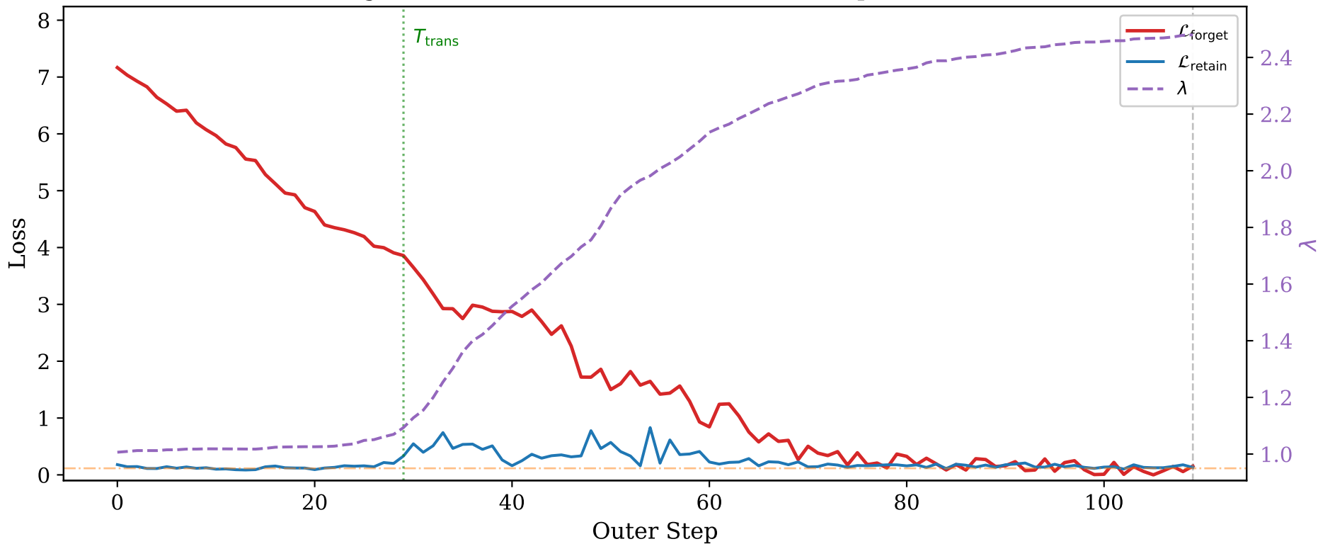
TOFU forget01 — Llama-3.2-1B: BLADE, 110 Steps (HM = 0.811)
