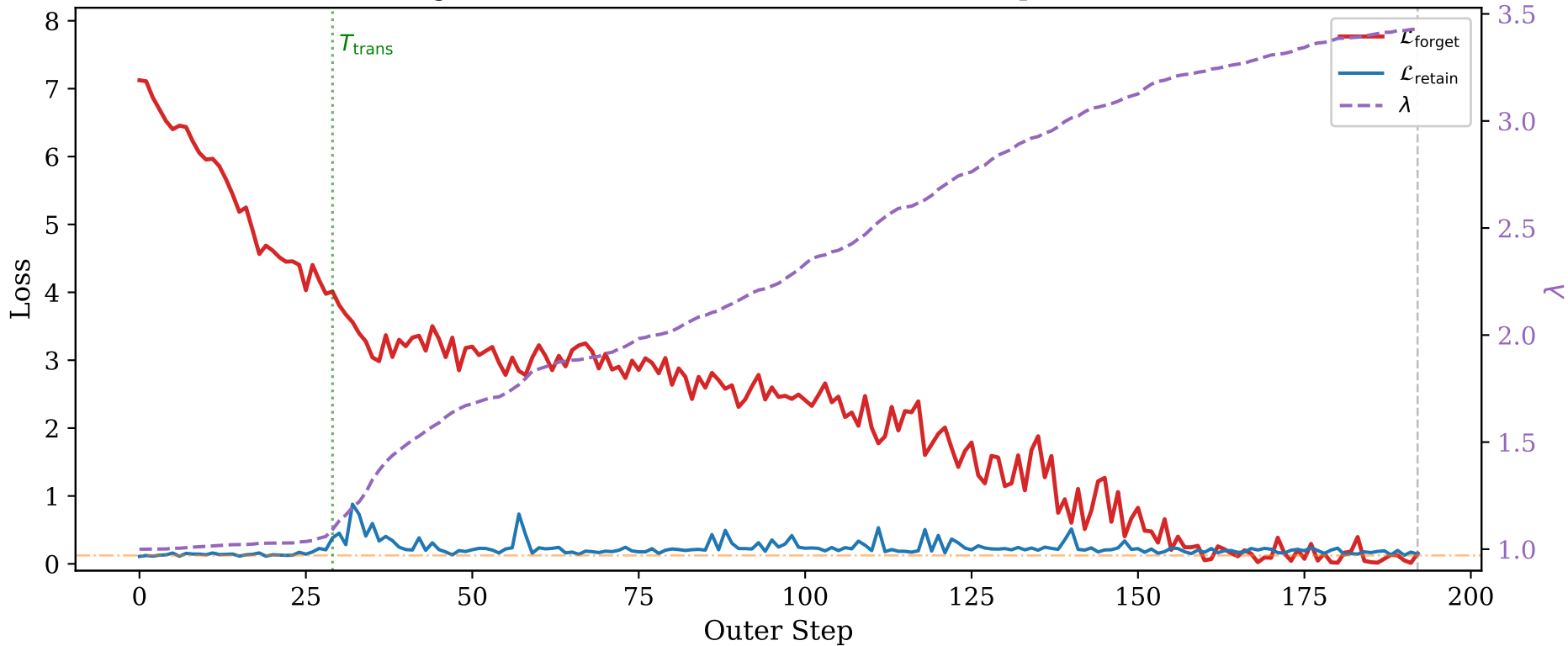
TOFU forget05 — Llama-3.2-1B: BLADE, 193 Steps (HM = 0.804)
