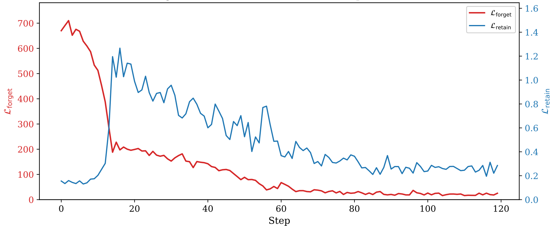
TOFU forget10 — Llama-3.2-1B: PDU, 120 Steps (HM = 0.797)
