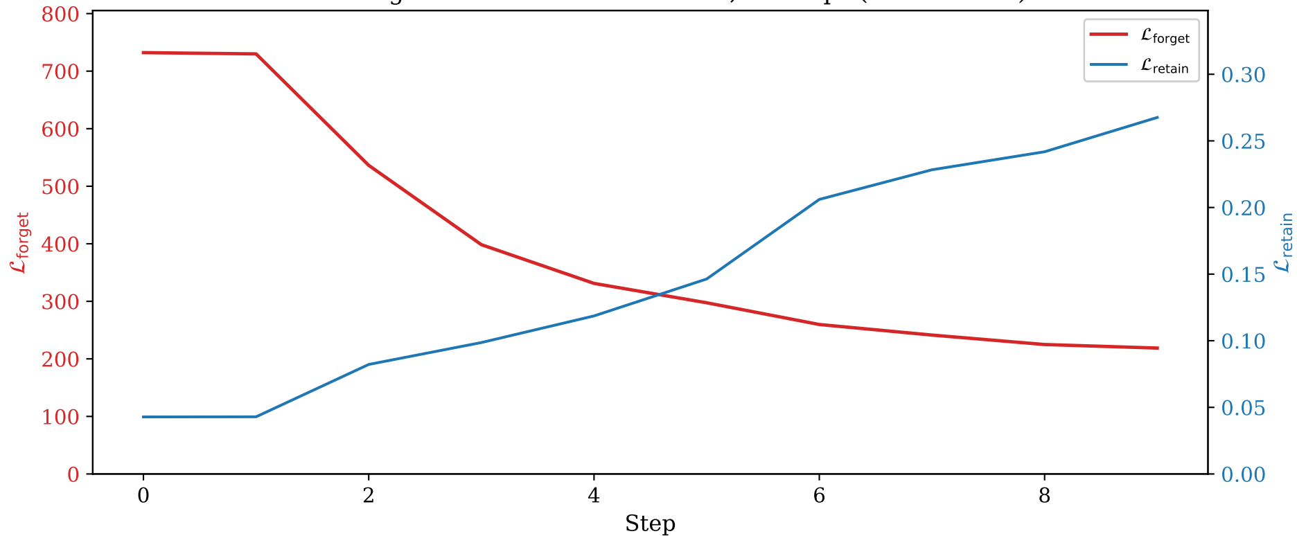
TOFU forget01 — Llama-3.2-3B: PDU, 10 Steps (HM = 0.742)
