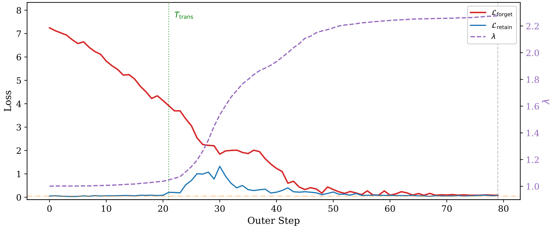
TOFU forget01 — Llama-3.2-3B: BLADE, 80 Steps (HM = 0.849)
