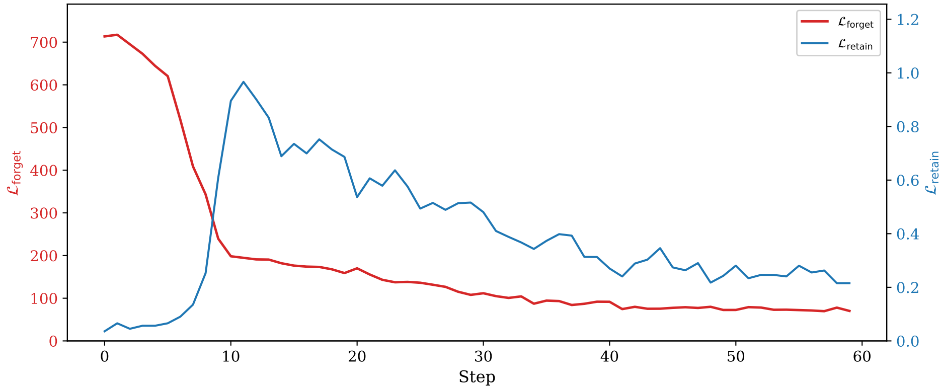
TOFU forget05 — Llama-3.2-3B: PDU, 60 Steps (HM = 0.843)
