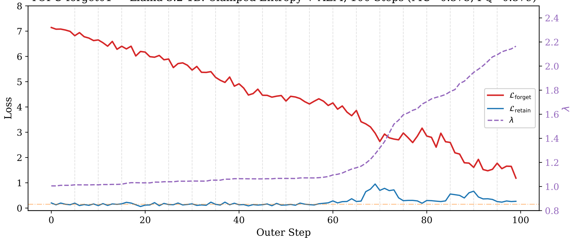
TOFU forget01 — Llama-3.2-1B: Clamped Entropy + ALM, 100 Steps (MU=0.575, FQ=0.579)
