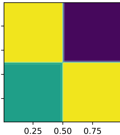
OEDG 2024
