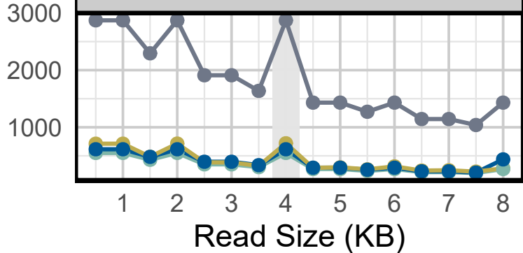
IOPS
