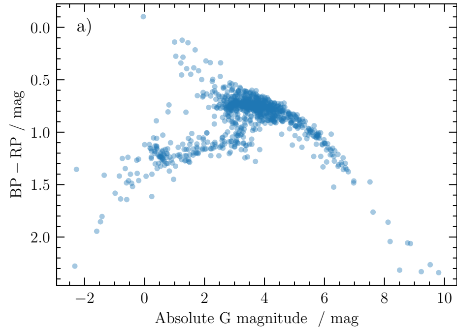
Gaia DR3
