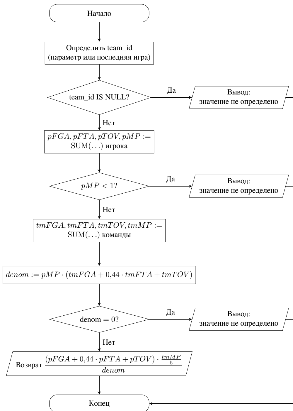
Рисунок 2.6 — Схема алгоритма вычисления функции calculate_usg
