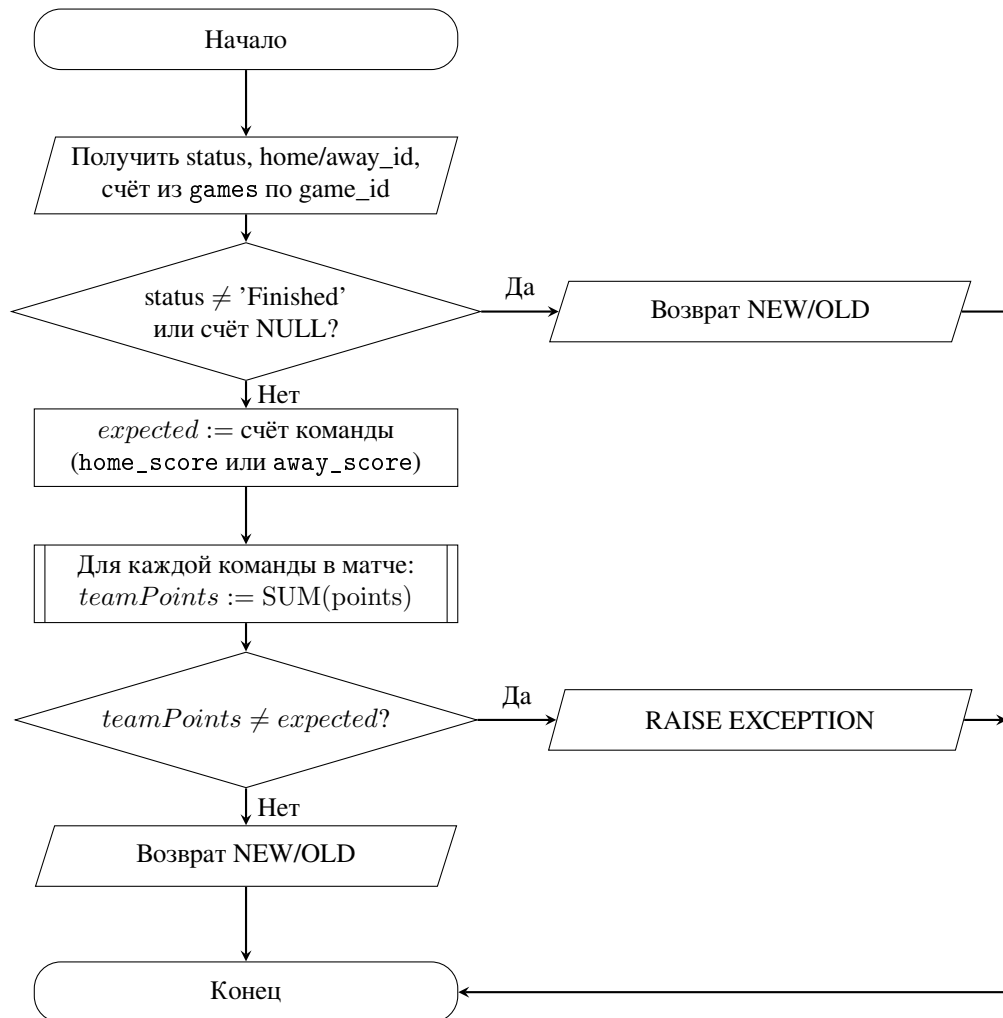
Рисунок 2.2 — Схема алгоритма функции-триггера trg_validate_team_score_row
