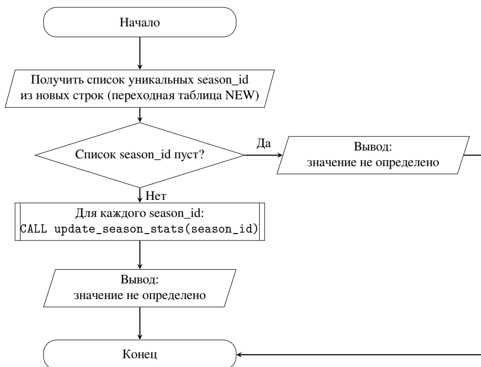
Рисунок 2.3 — Схема алгоритма функции-триггера trg_update_season_stats_func
