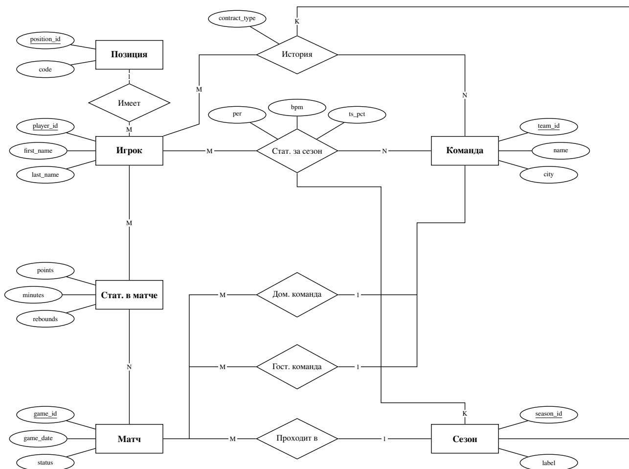
Рисунок 1.1 — Концептуальная ER-диаграмма в нотации Чена
