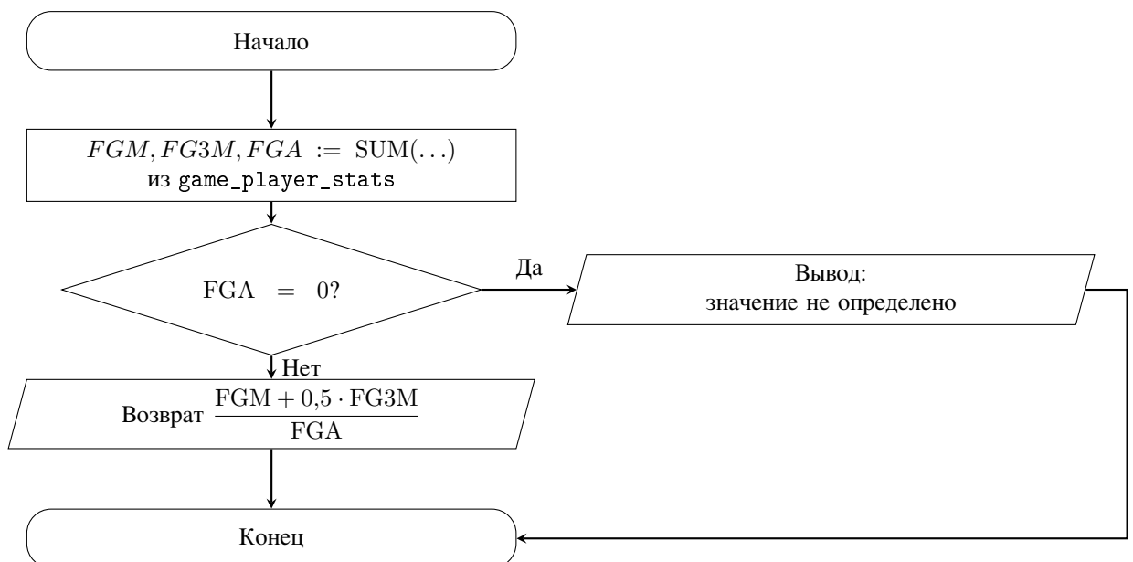
Рисунок 2.5 — Схема алгоритма вычисления функции calculate_efg
