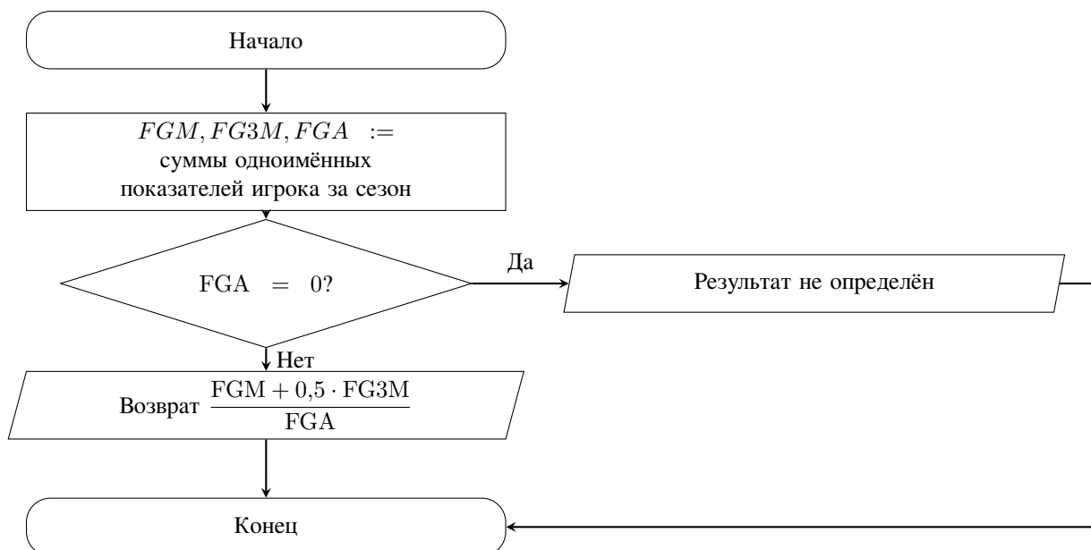
Рисунок 2.5 — Схема алгоритма вычисления функции calculate_efg
