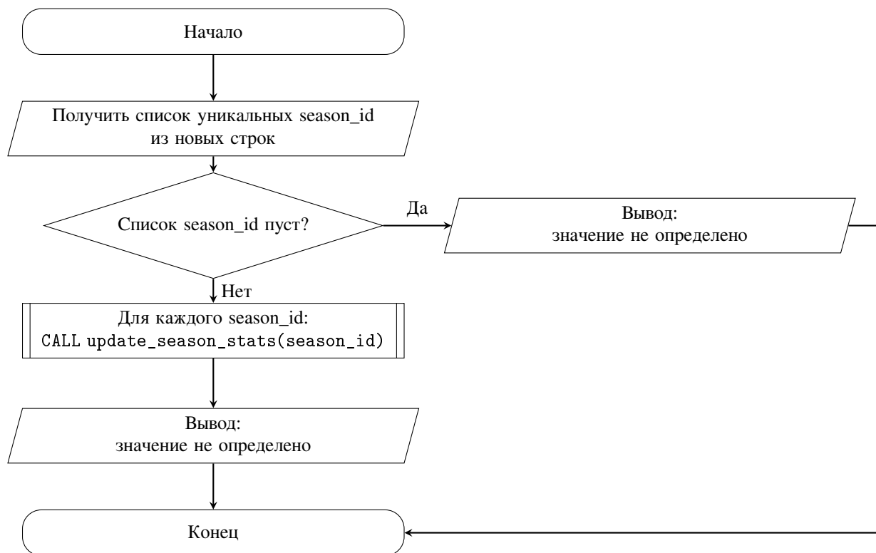
Рисунок 2.3 — Схема алгоритма функции-триггера trg_update_season_stats_func
