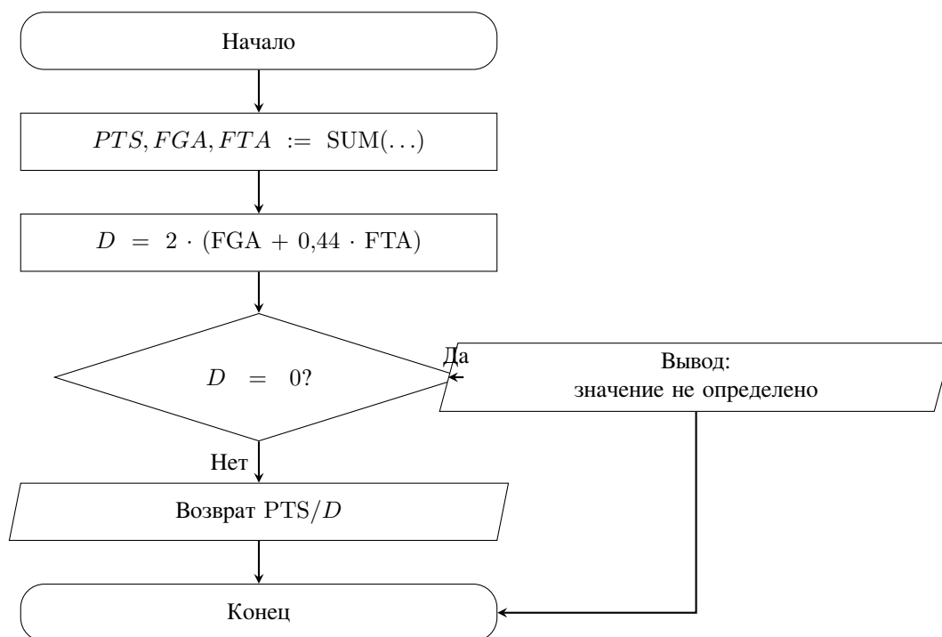
Рисунок 2.4 — Схема алгоритма вычисления функции calculate_ts
