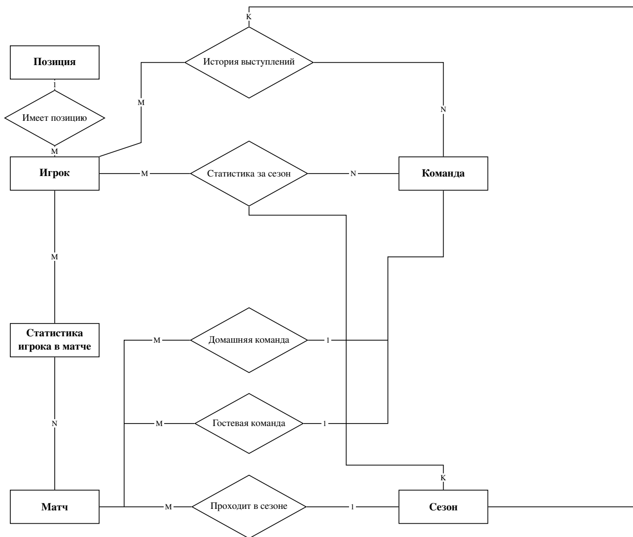
Рисунок 1.1 — Концептуальная ER-диаграмма в нотации Чена
