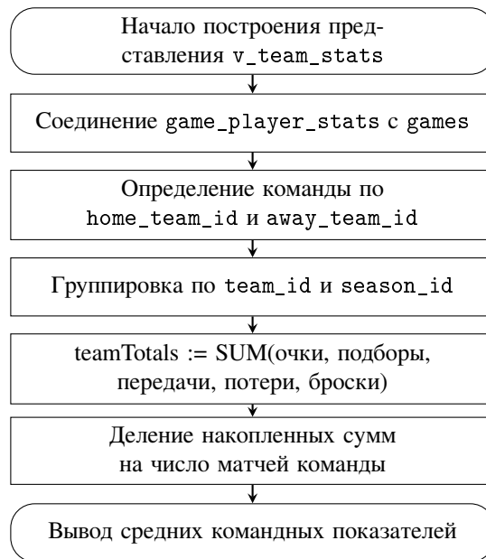
Рисунок 2.9 — Схема алгоритма агрегирования командной статистики в представлении v_team_stats
