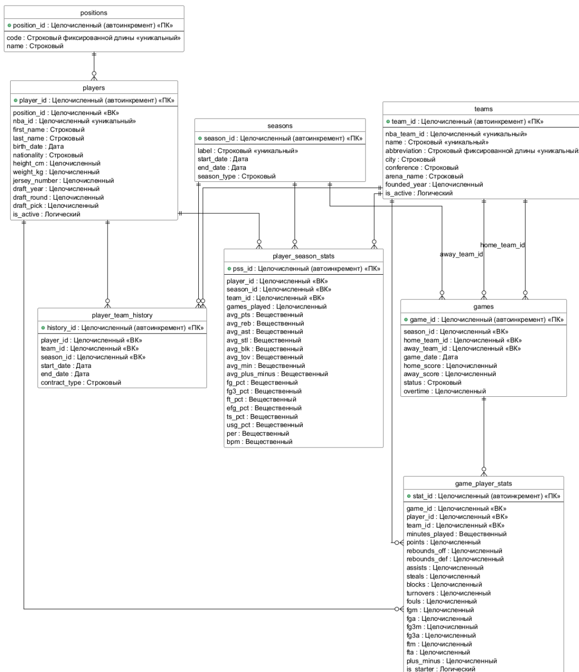
Рисунок 2.1 — Схема реляционной базы данных
