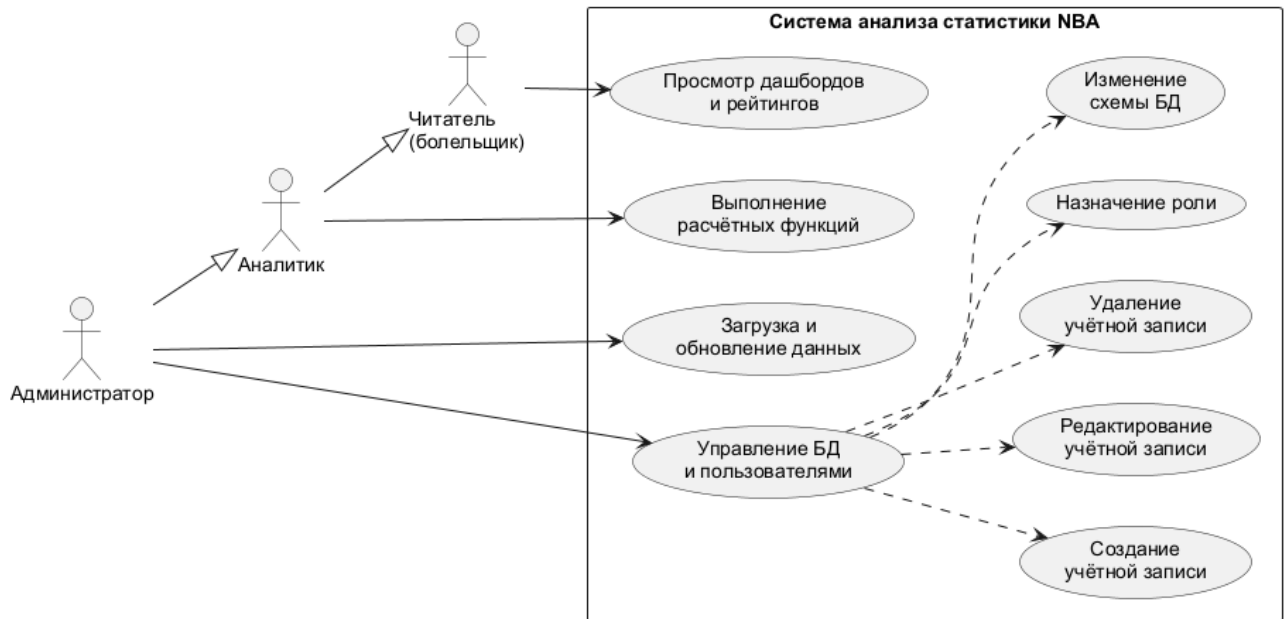
Рисунок 1.2 — Диаграмма вариантов использования
