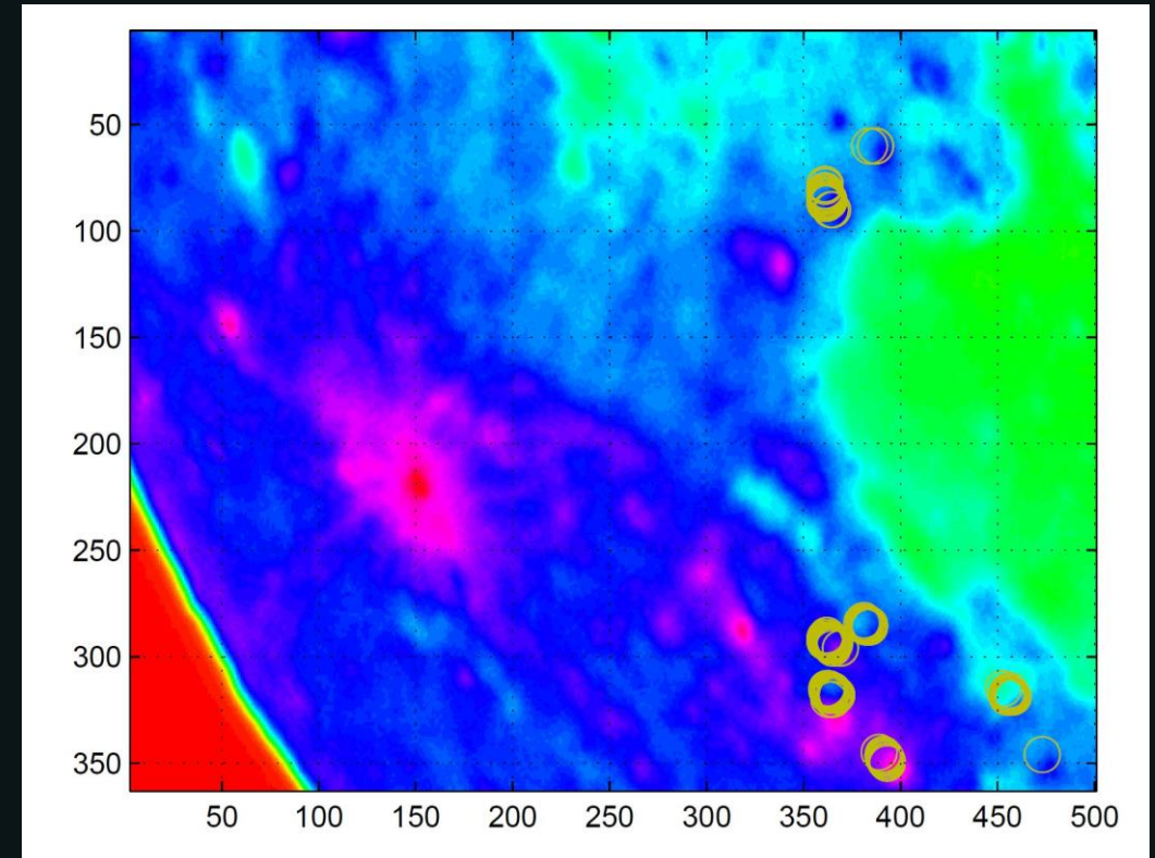
B. "Ηπειρωτικά" UFOs (σε σχήμα δίσκου): Κινούνται πάνω από την επιφάνεια της Σελήνης. Μέγεθος: Διάμετρος περίπου 25 έως 40 km . Αναφέρεται ταχύτητα έως 40000-115000 km/h .
