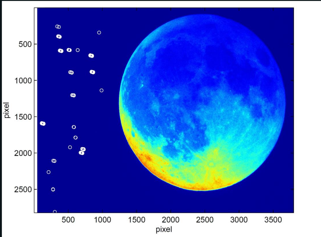
A. "Ατμοσφαιρικά" UFOs: Φαίνονται σχετικά ακίνητα , κινούνται συγχρονισμένα με τη Σελήνη. Μέγεθος από 440 μέτρα έως 1.800 μέτρα . Παρουσιάζουν αναλαμπές διάρκειας 100-500 ms.
